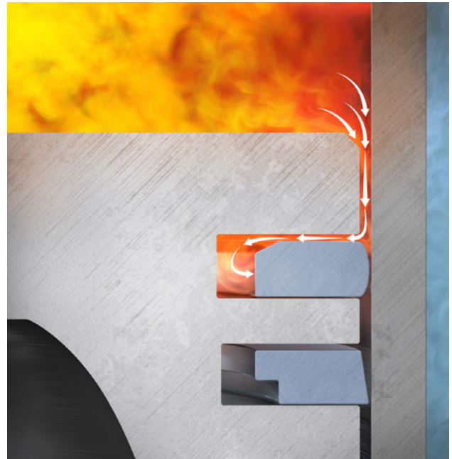
Abdichtung von Verbrennungsgasen
