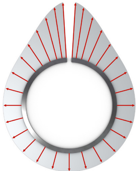
Abb. 3: positiv-ovale Radialdruck- verteilung
