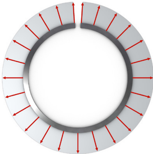
Abb. 2: symmetrische Radial- druckverteilung
