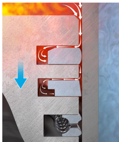
Abb. 6: mit Verbrennungsdruck
