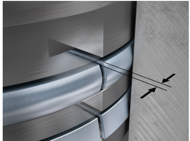
Abb. 1: Stoßspiel im eingebauten Zustand
