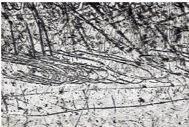
Abb. 4 und 5: Beispiele für Rollspuren an der oberen Ringflanke
