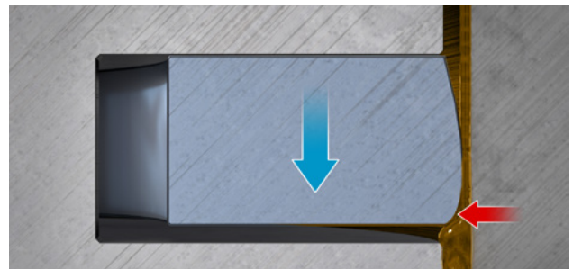
Abb. 5: schwaches Aufschwimmen in der Abwärtsbewegung
