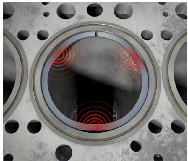
Abb. 3: Abheben des Kolbenrings von der Lauffläche
