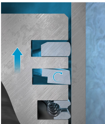
Abb. 5: ohne Verbrennungsdruck
