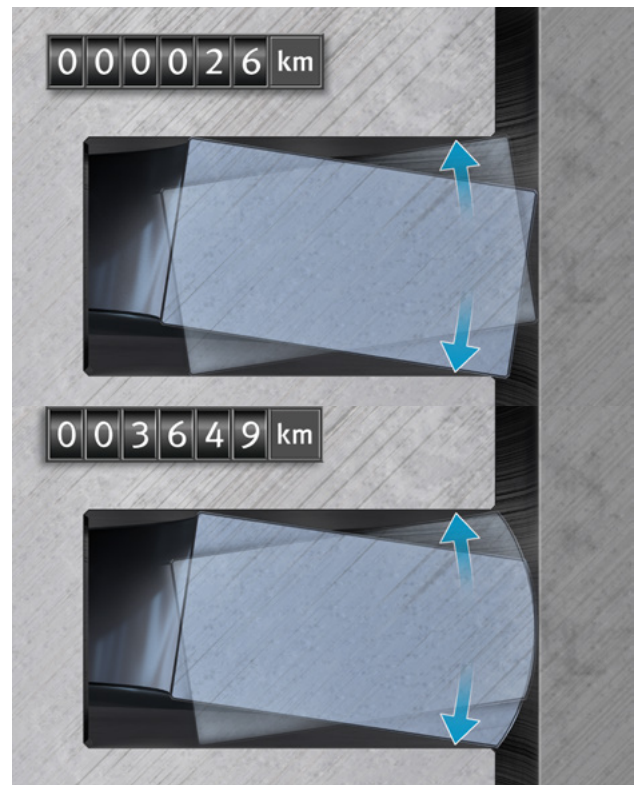
Abb. 1: Balligkeit durch Einlaufverschleiß
