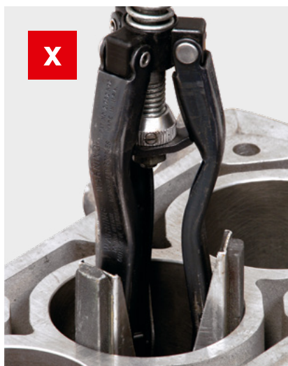
Abb. 2: federbelastete Honsteine
