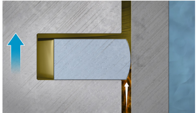
Abb. 1: Abdichtung durch Nutenflanke
