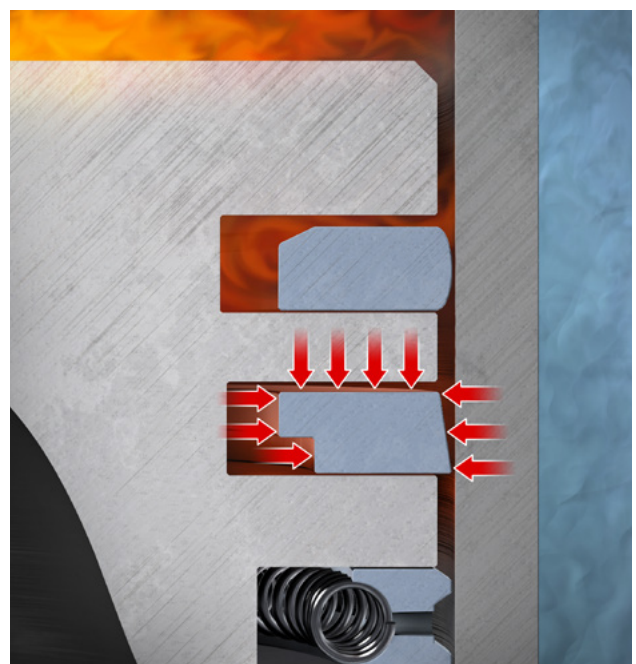
Gasdruck am Minutenring
