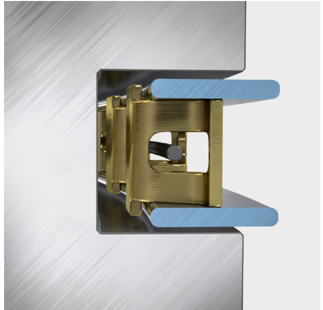
Dreiteiliger Ölabstreifring
