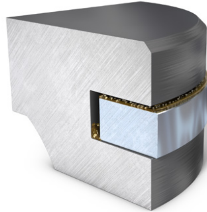
Abb. 2: Schmutz- und Ölablagerungen in der Ringnut verbinden sich zu einer Schleifpaste.
