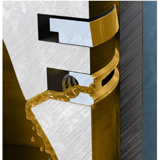
Öl abstreifen und verteilen
