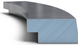
Minutenring mit Innenwinkel unten
