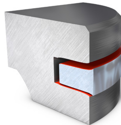
Abb. 3: Kolbenringnuterweiterung durch heruntergeschliffenen Kolbenring
