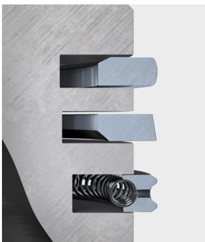
Abb. 2: Kolbenringe ungespannt – Vertwistung noch unwirksam
