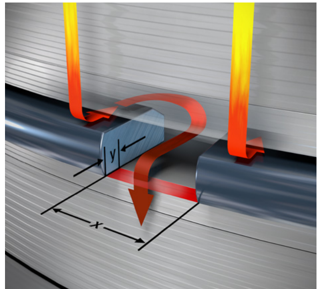
Abb. 4: Drosselfenster
