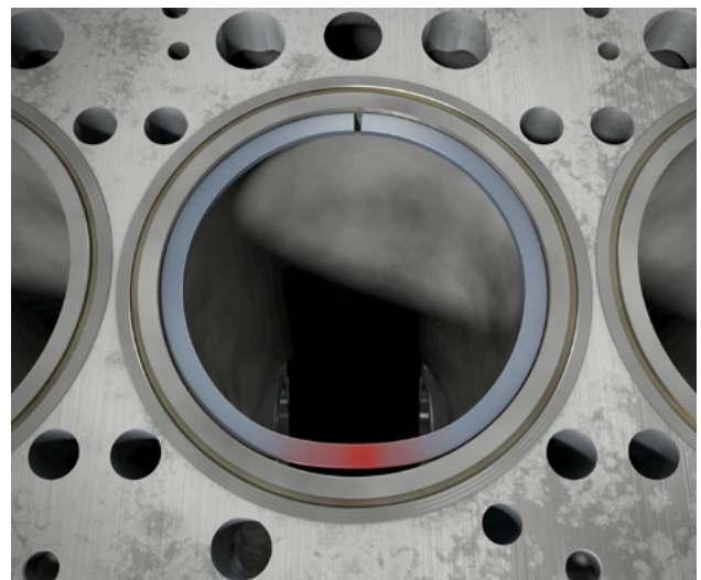
Abb. 2: Bildung von Sichelspalten durch übermäßiges Aufspreizen
