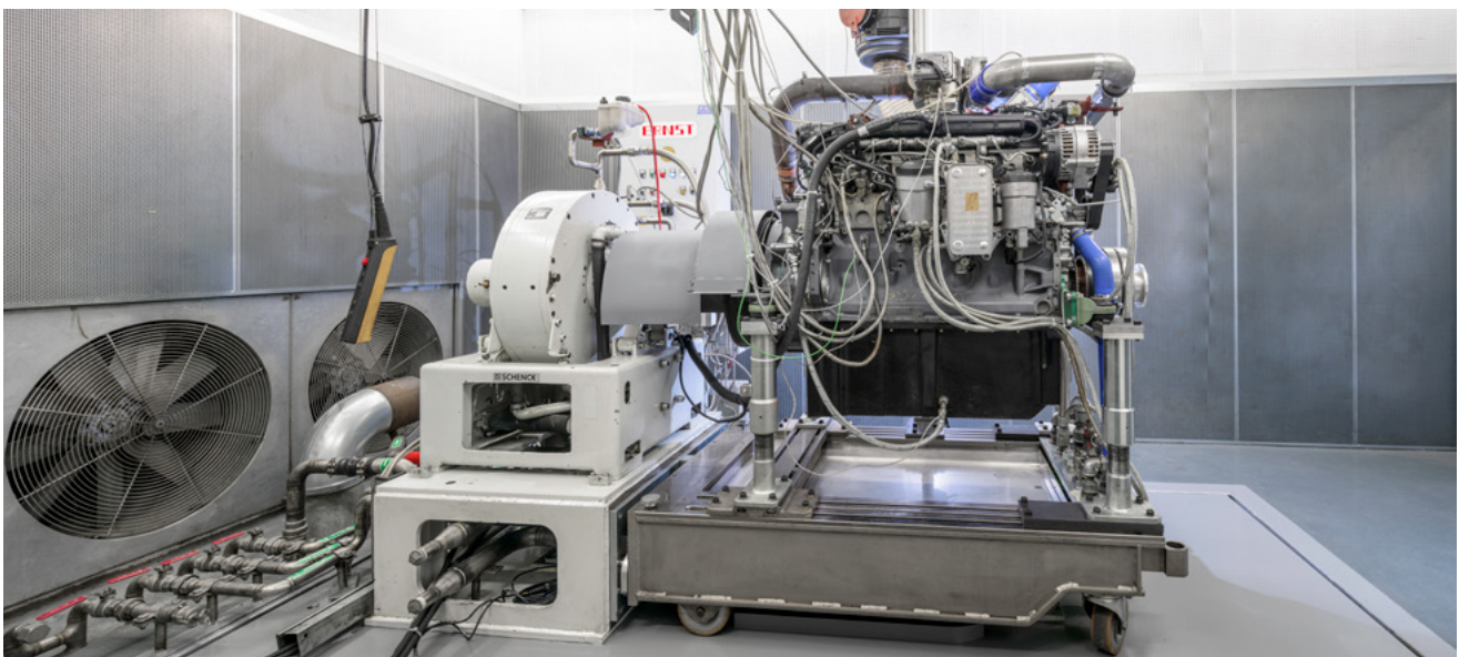
Einlauf- und Verschleißtests auf dem Motorenprüfstand
