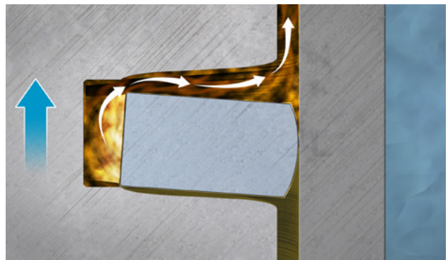
Abb. 3: Verdichtungstakt
