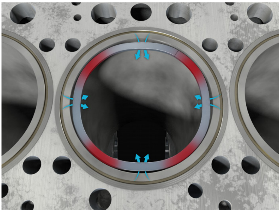
Abb. 1: schlechtes Formfüllungsvermögen
