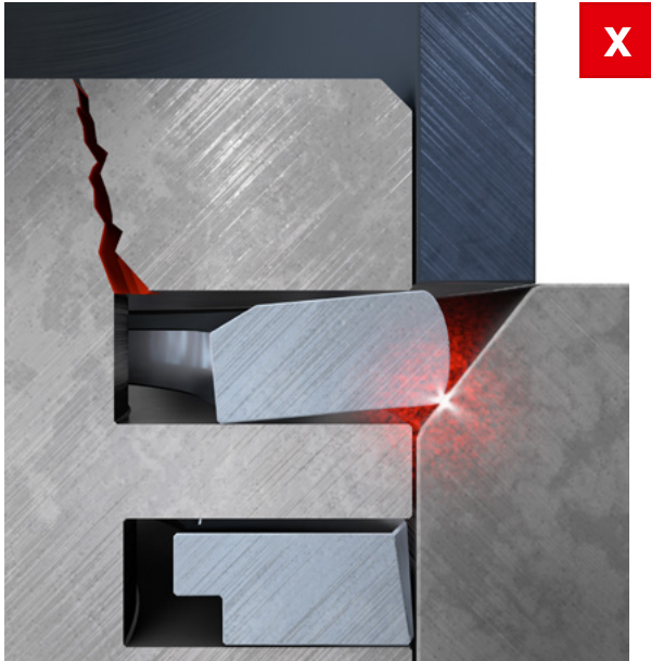
Abb. 1: zu große Fase an der Zylinderbohrung – der Kolbenring federt bei der Montage zwischen Kolbenringspannband und Zylinder aus und der Kolben blockiert
