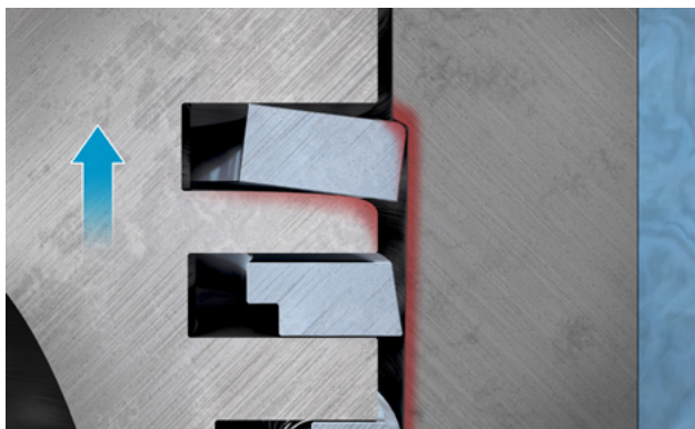
Abb. 2: Anschlagen des Kolbenrings bei altem Kolben
