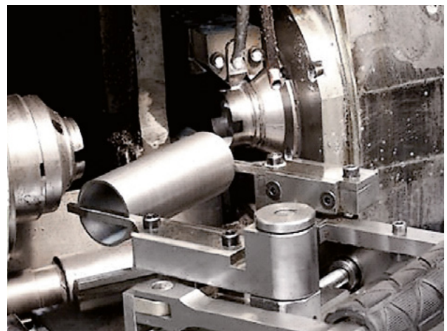
Drehmaschine zur Laufflächenbearbeitung
