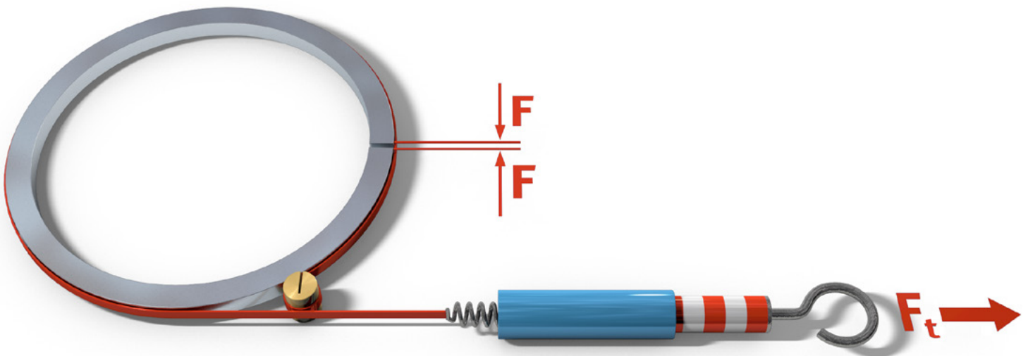
Abb. 1: Tangentialkraftmessung
