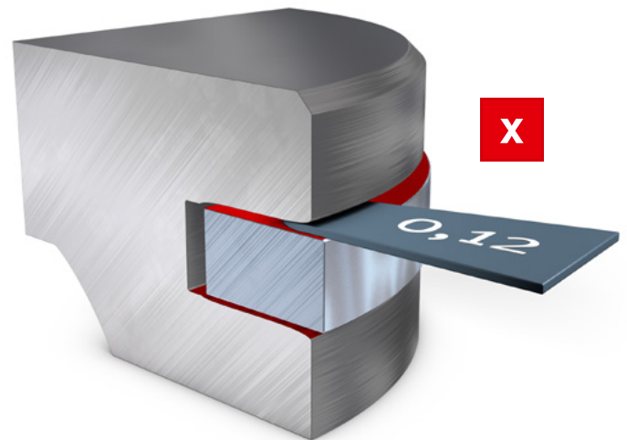
Abb. 2: verschlissene Ringnut
