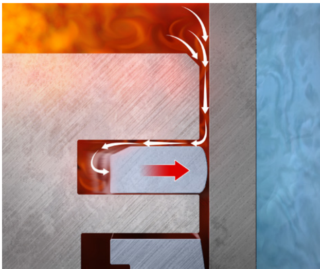
Abb. 1: Anpressdruckverstärkung
