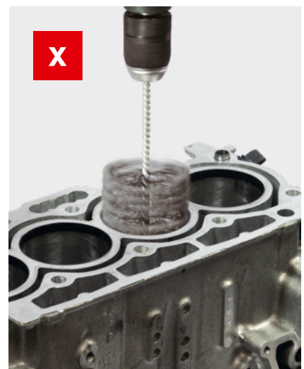
Abb. 3: Honbürsten
