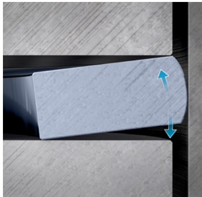
Ringvertwüstung
